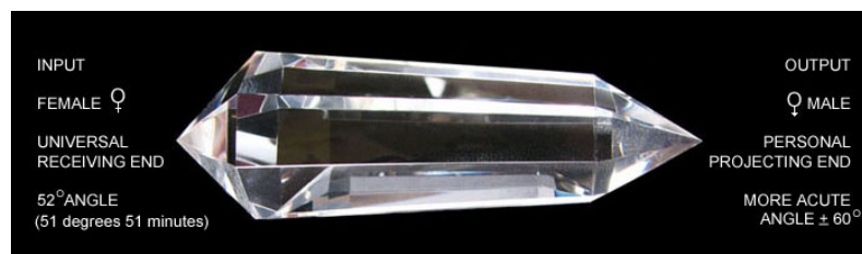
VOGEL CRYSTAL
